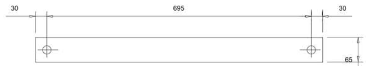
ITEM 4 TIE STRAP 65 x 8 FLAT BAR 755 LONG
